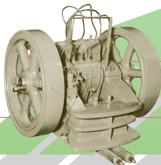
SJ15ブレーキクラッシャ／昭和30年
