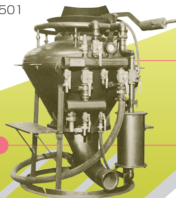
グッドマン（コンクリート圧送機）／昭和41年
